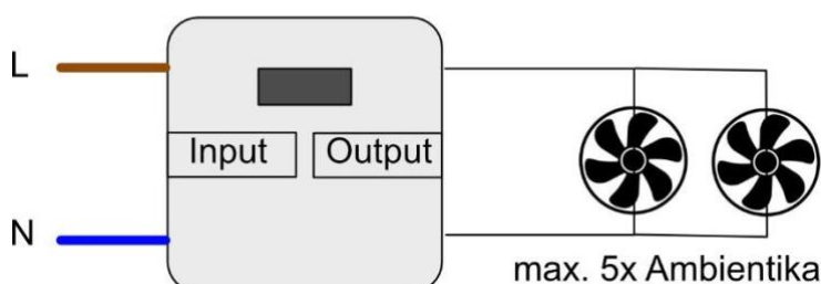
Betriebsstundenzähler
